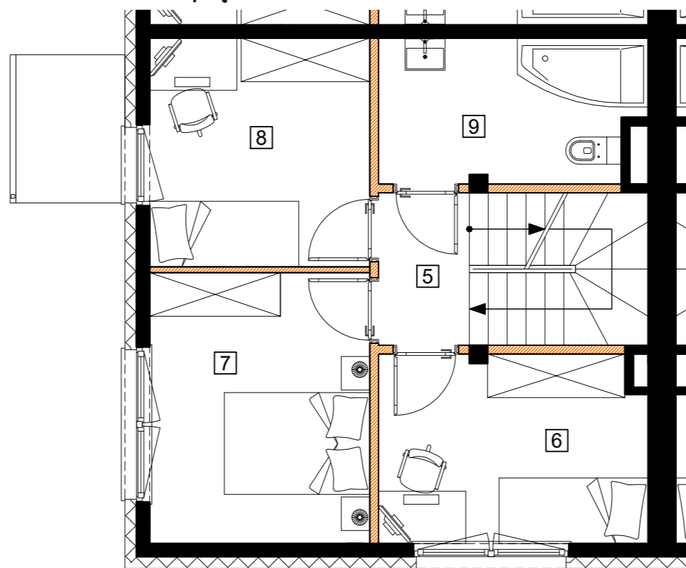
Rzut piętra
