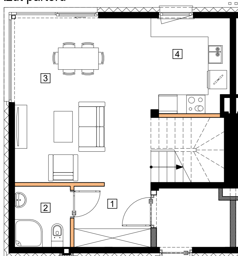
Rzut parteru
