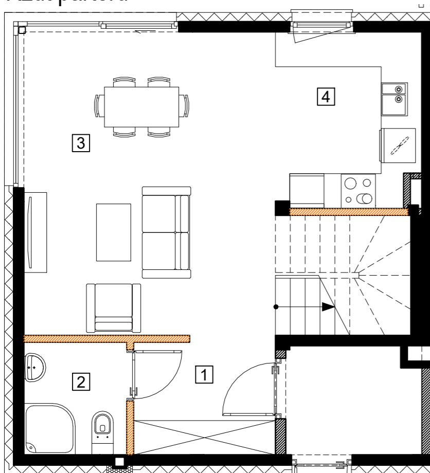
Rzut parteru
