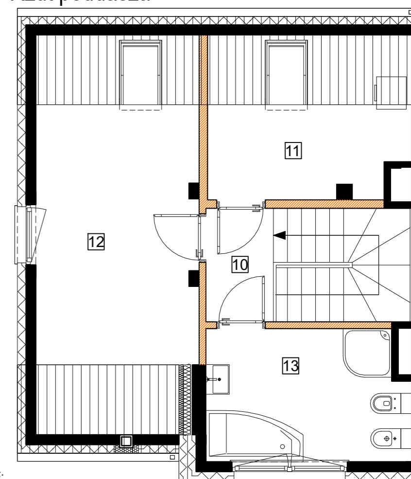
Rzut poddasza
