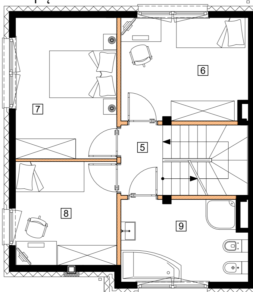
Rzut piętra
