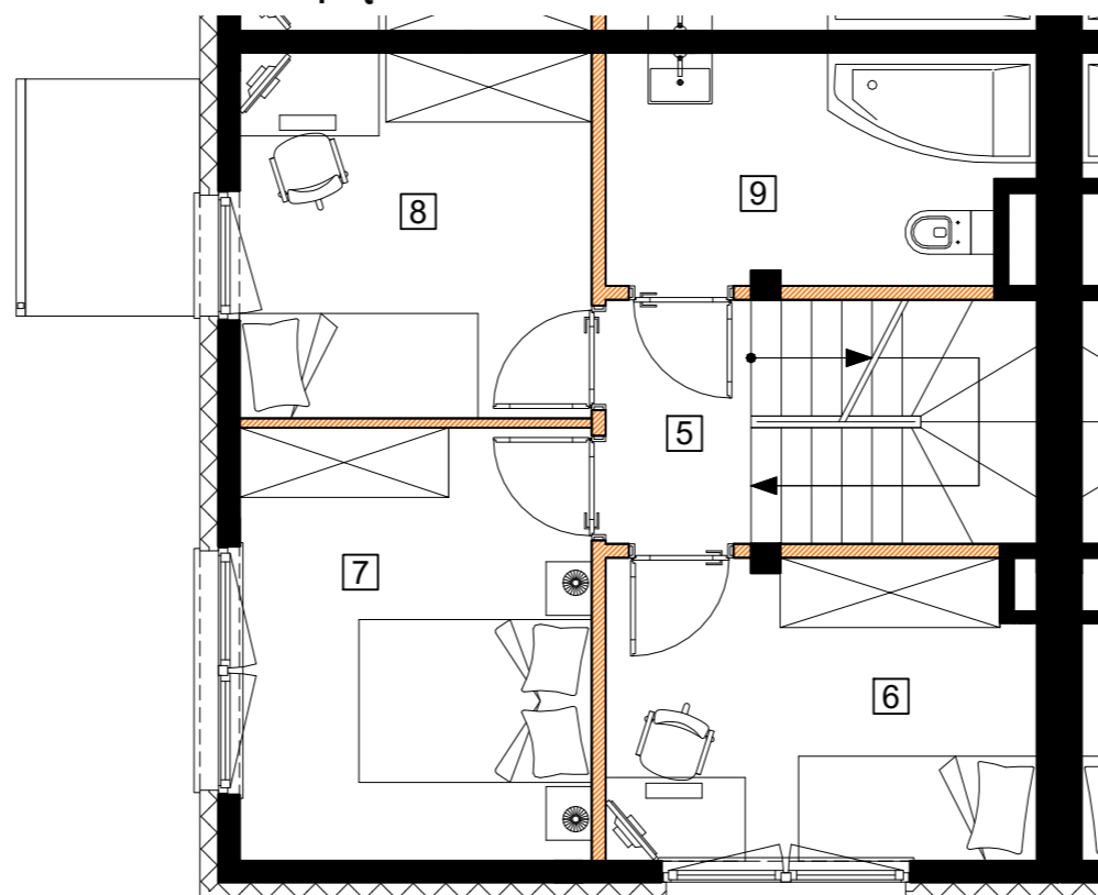
Rzut piętra
